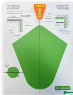
Gabarit de perçage pour les raccords de WC
