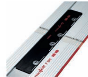
Verbindungsstück F-VS Verbinder von Führungs- schienen Führungsschienen- System Art. Nr. 464805
